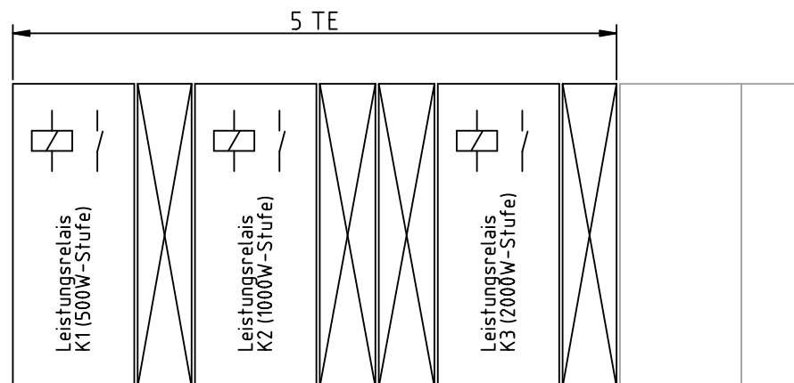
Variante 2: Anreihung links an weitere Einbaugeräte
