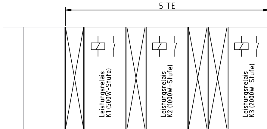
Variante 1: Anreihung rechts an weitere Einbaugeräte
