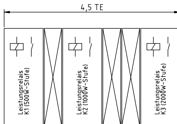
Variante 3: beidseitig freier Einbau
